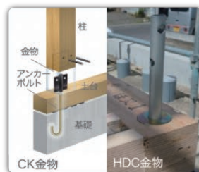
■JWOOD 工法の接合部（柱と基礎）
