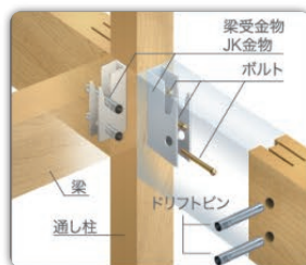
■JWOOD 工法の接合部（通し柱と梁）
